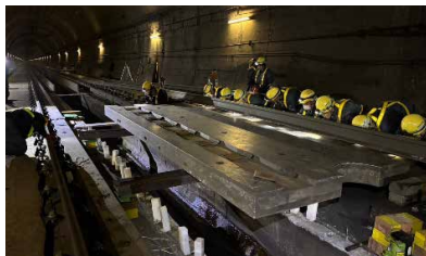
【スラブ低下工事状況】
